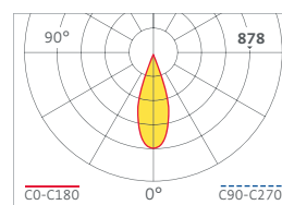
7W – 4000K – 38°
