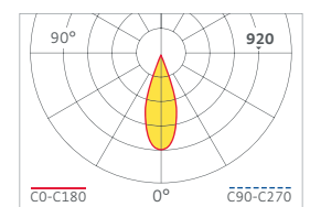
7W – 5000K – 38°
